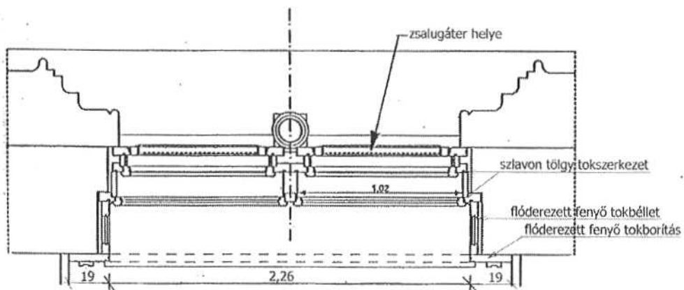
B-B metszet
