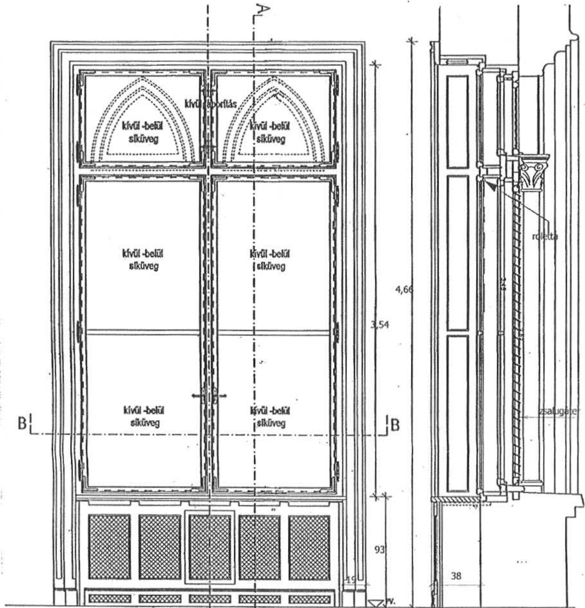
Belső nézet
